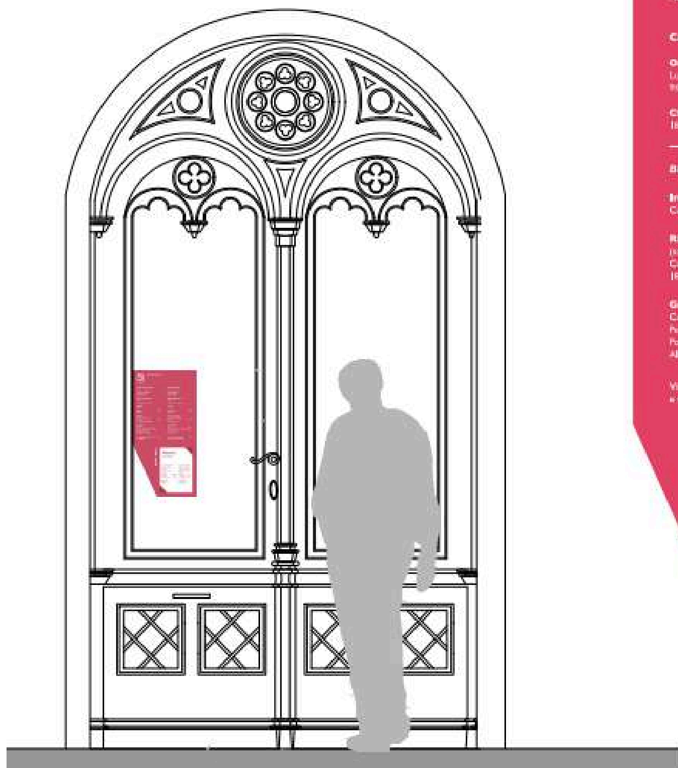
Prospetto _vista dall'esterno
