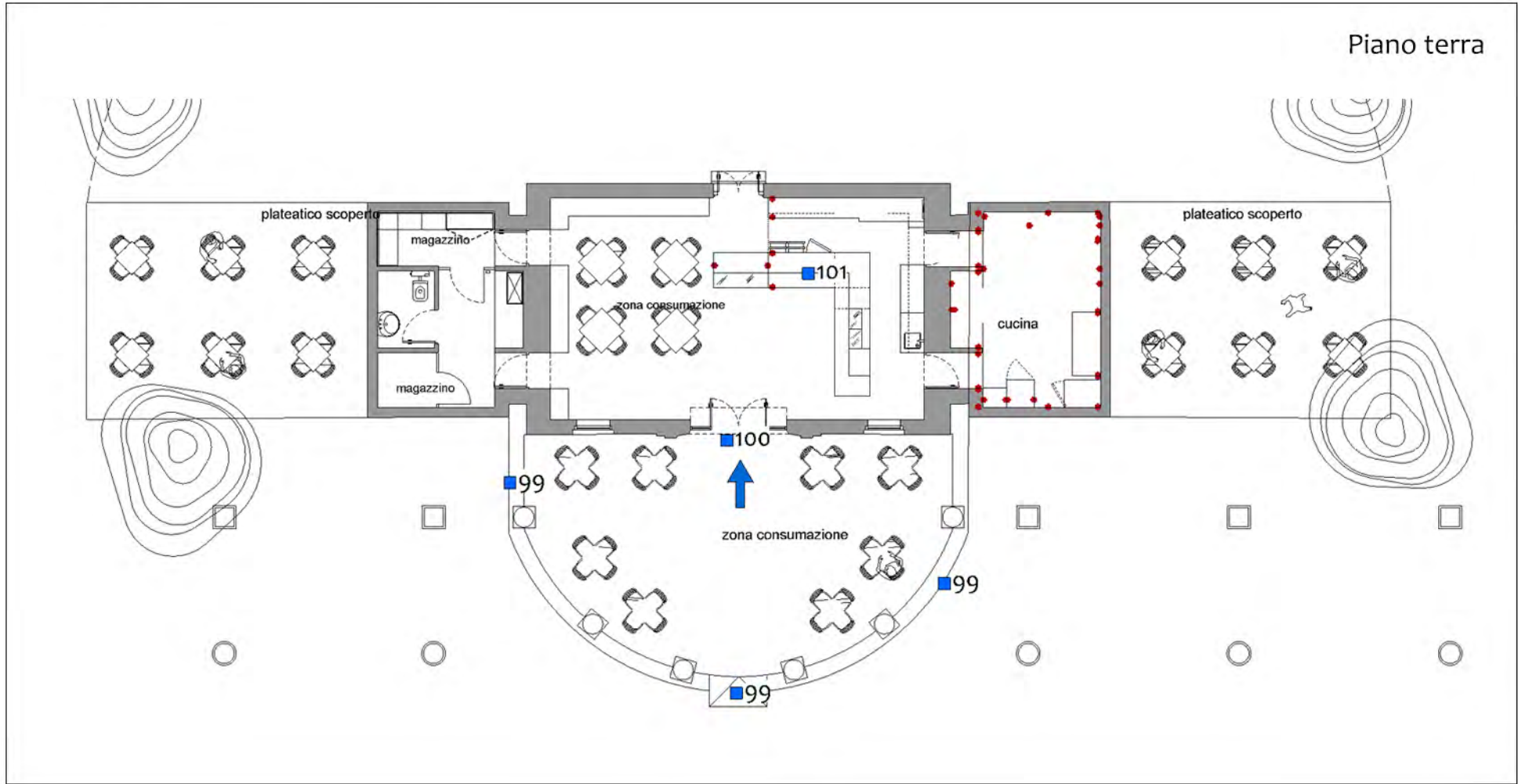
KAFFEEHAUS_PLANIMETRIA GENERALE non in scala
